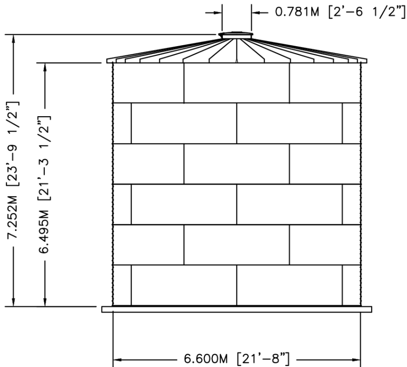
ELEVATION
